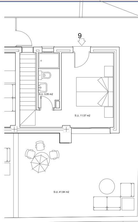
PLANTA ATICO
