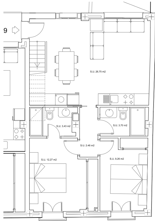
PLANTA PRIMERA
